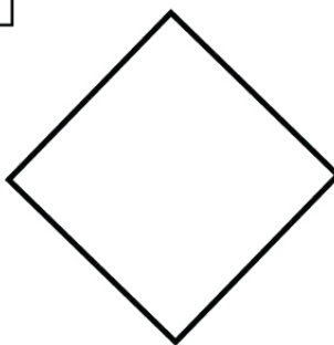
Rhombus
